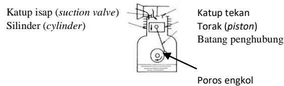
Gambar 1. Diagram kompresor
