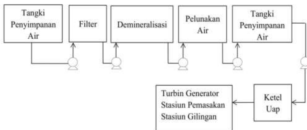
Gambar 2.1 Sistem Kerja Air Umpan Ketel UAP
